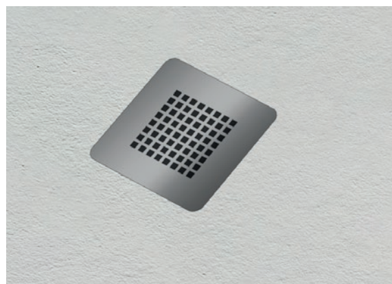
Evacuation : diamètre 90 mm, grille en inox poli, possible en blanc ou anthracite en option
